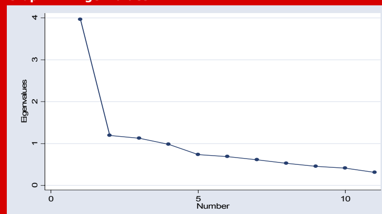
Graph 1 Eigenvalues
